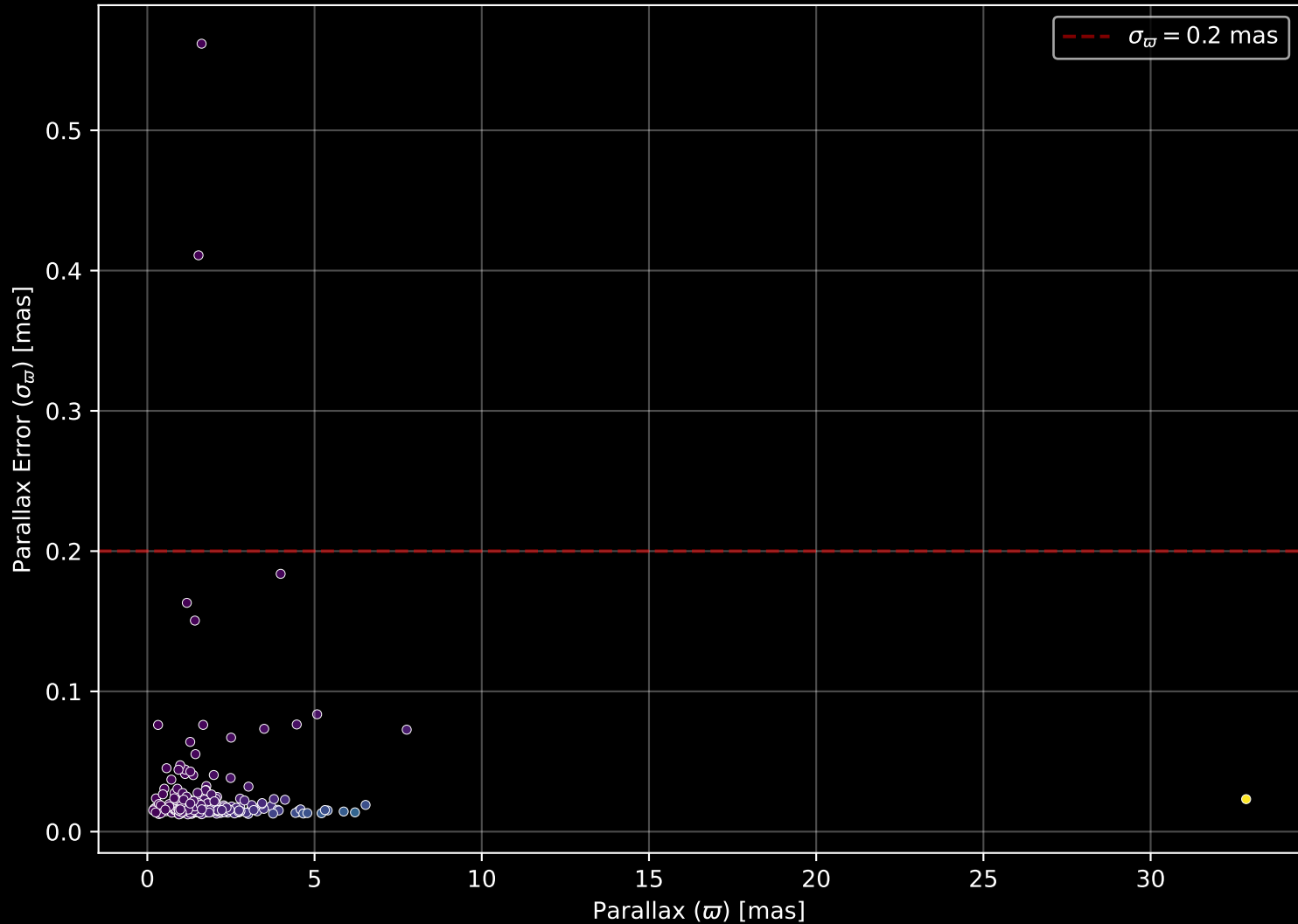
GALAH DR4 Field: [827] Parallax Quality (n= 286)
