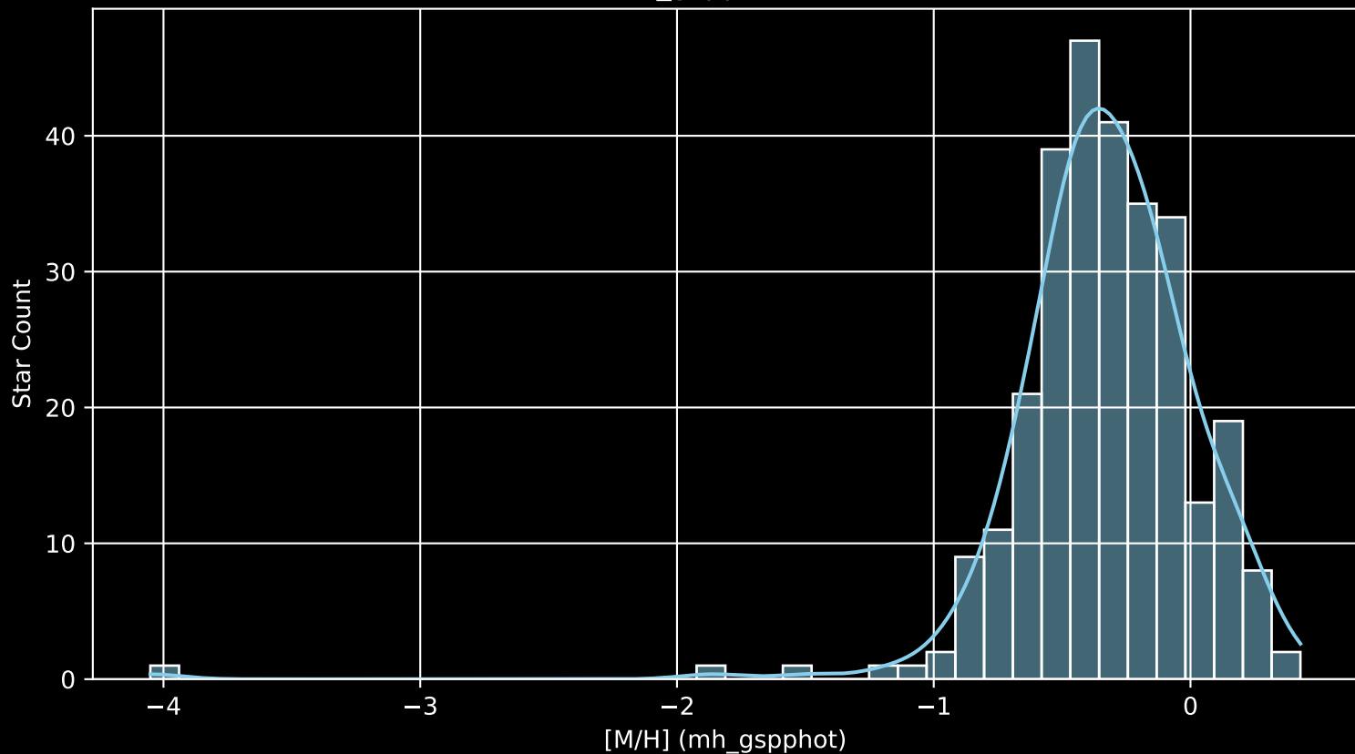
GALAH DR4 Field: [827] [M/H] (mh_gspphot) (n= 286)
