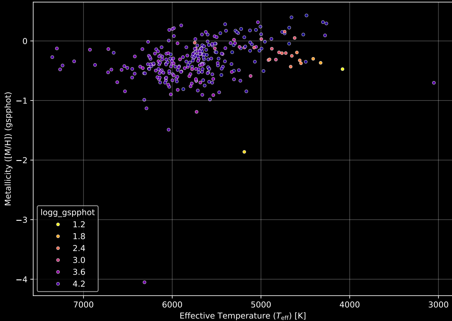
GALAH DR4 Field: [827] Stellar Population Parameters (n= 286)
